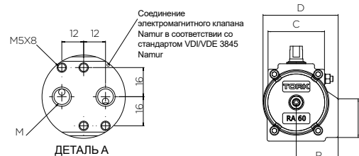
Нижнее соединение привода (шаровые, поворотные дисковые затворы, запорный клапан) в соответствии со стандартом ISO/DIN 3337
