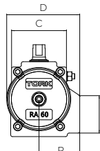
Нижнее соединение привода (шаровые, поворотные дисковые затворы, запорный клапан) в соответствии со стандартом ISO/DIN 3337
