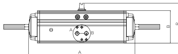
Верхнее соединение привода (коробка переключателя, позиционер) в соответствии со стандартом VDI/VDE 3845
